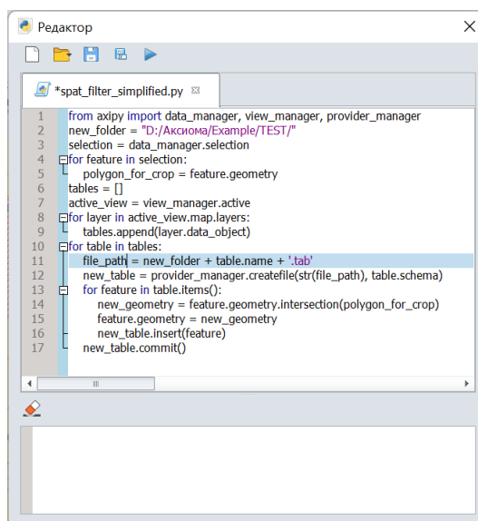
Рисунок 113 – Окно редактора кода
