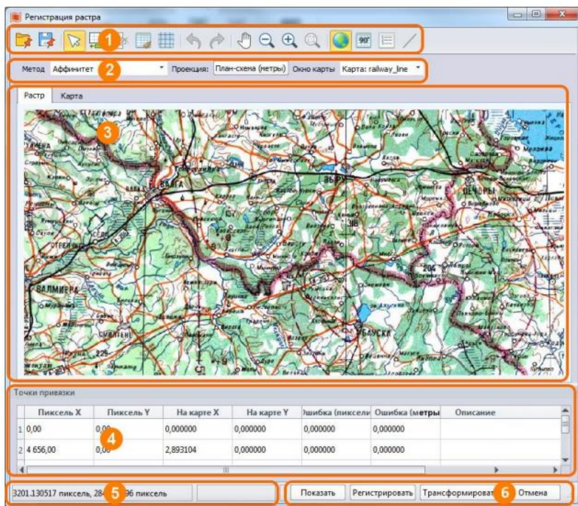
Рисунок 83 - Окно регистрации растра
