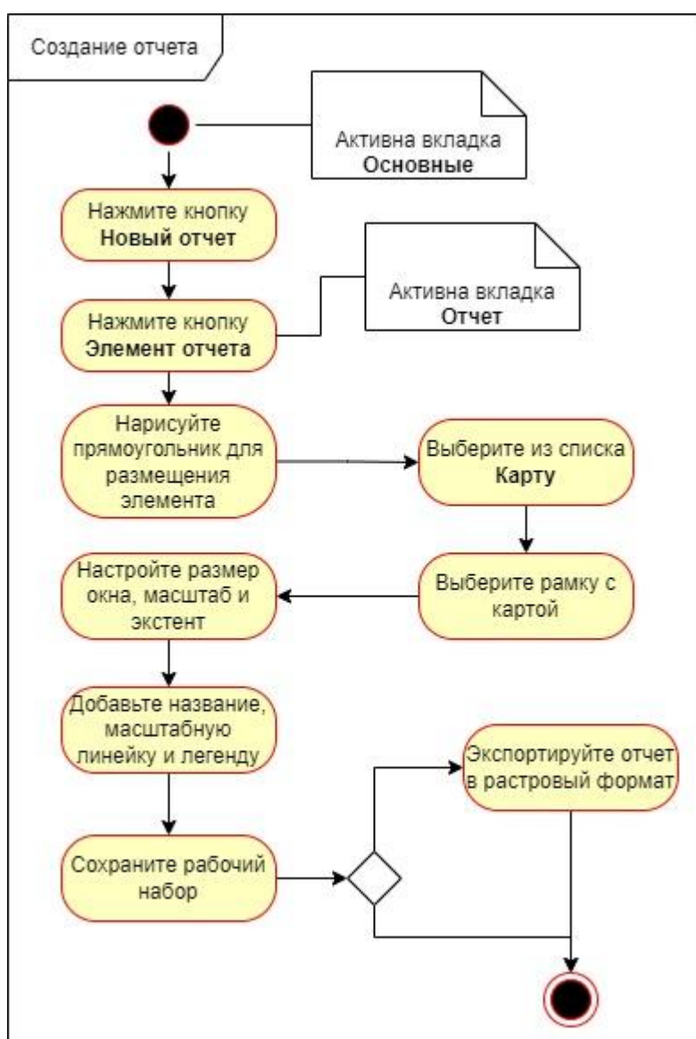
Рисунок 42 – Последовательность работ по созданию отчета
