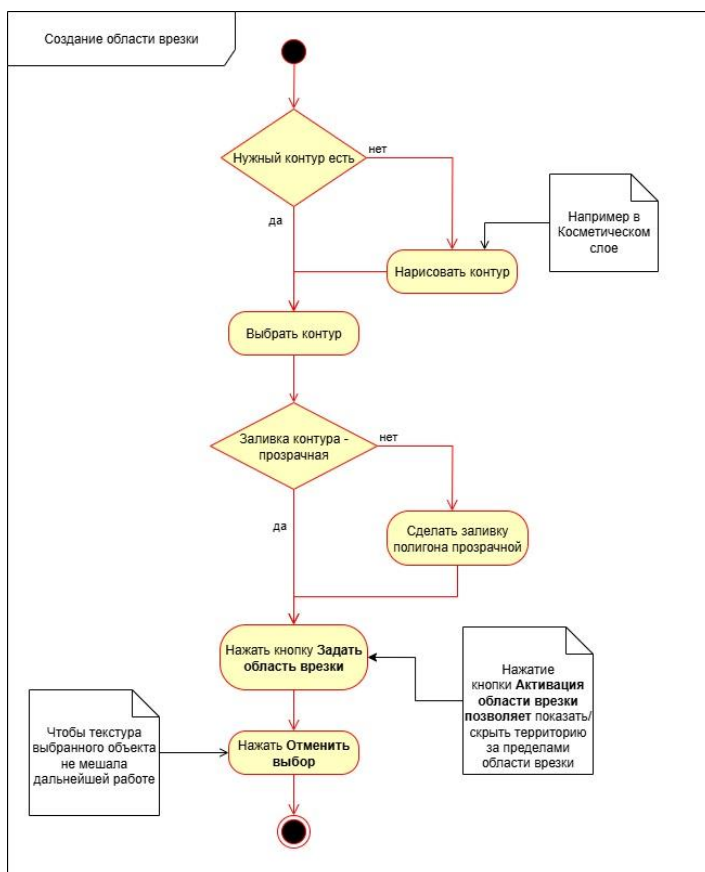
Рисунок 35 - Последовательность действий для создания области врезки.
