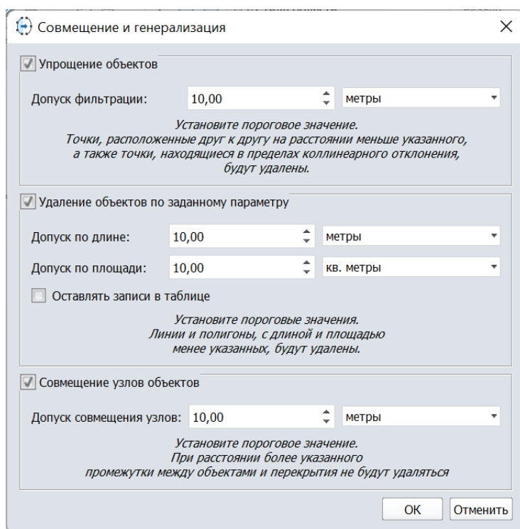
Рисунок 104 - Окно инструмента Совмещение и генерализация
