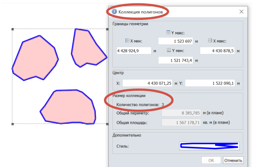
Рисунок 52 – Коллекция полигонов
