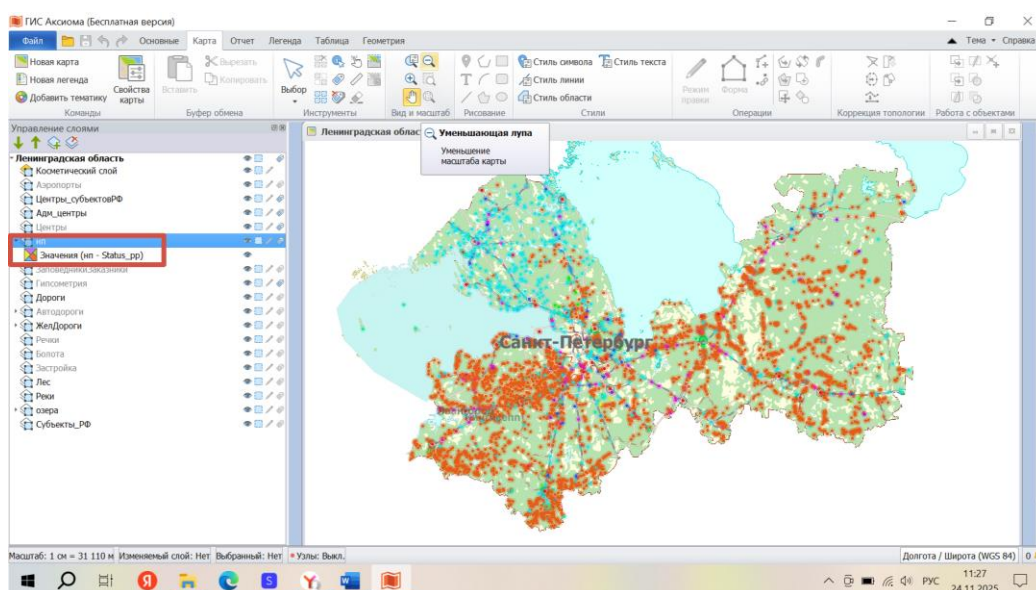
Рисунок 28 - Тематическая карта
