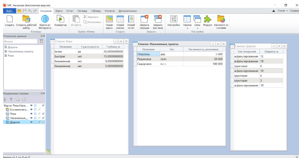
Рисунок 16 – Атрибутивные таблицы
