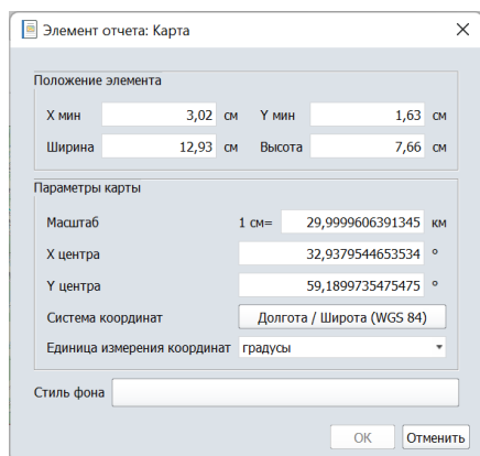
Рисунок 39 - Окно свойств элемента отчета
