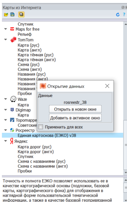
Рисунок 61 – Панель Карты из Интернета и окно добавления карт из интернета
