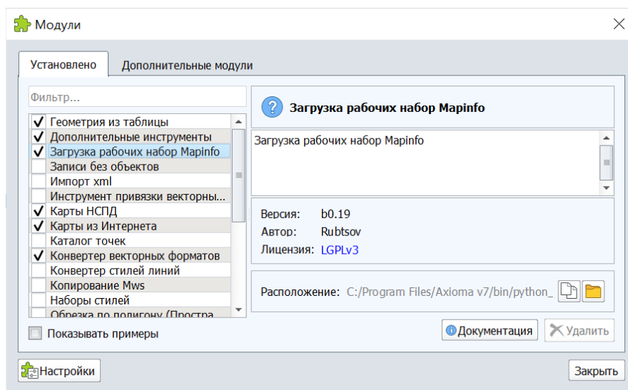
Рисунок 15 – Активация модуля Загрузка рабочих наборов MapInfo
