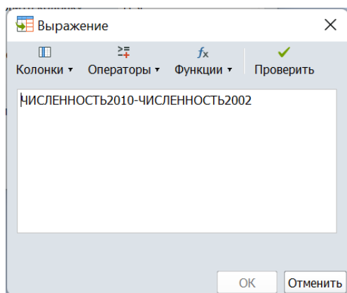
Рисунок 107 – Окно Выражения
