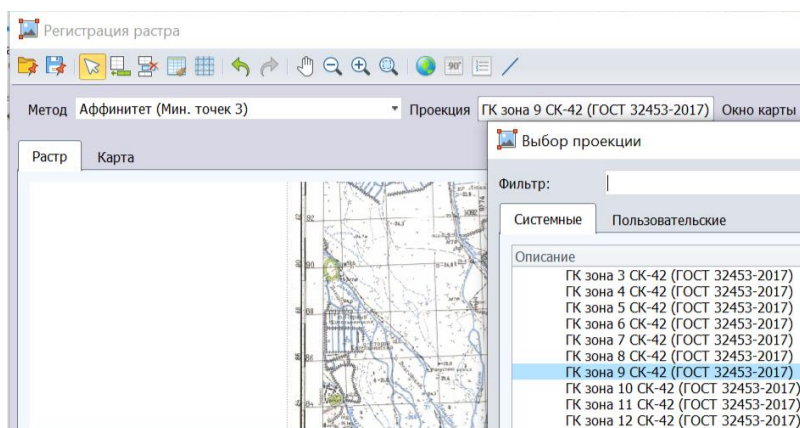
Рисунок 84 - Задание проекции
