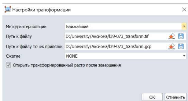
Рисунок 96 - Настройки трансформирования
