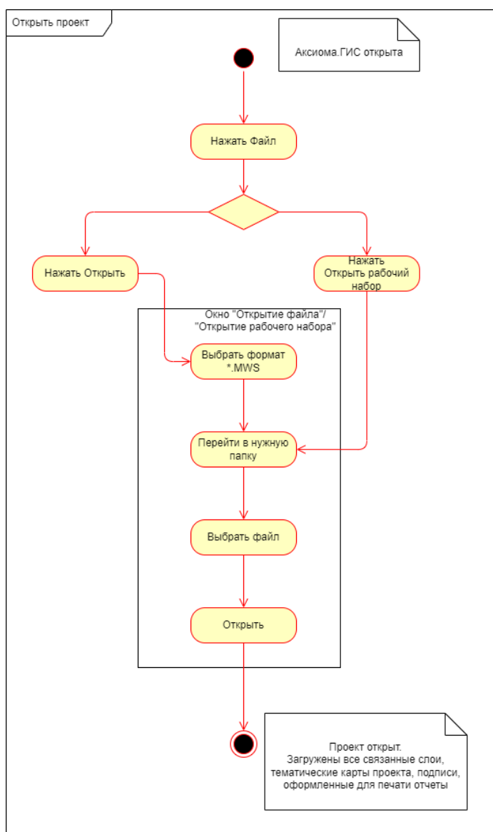
Рисунок 14- Загрузка проекта
