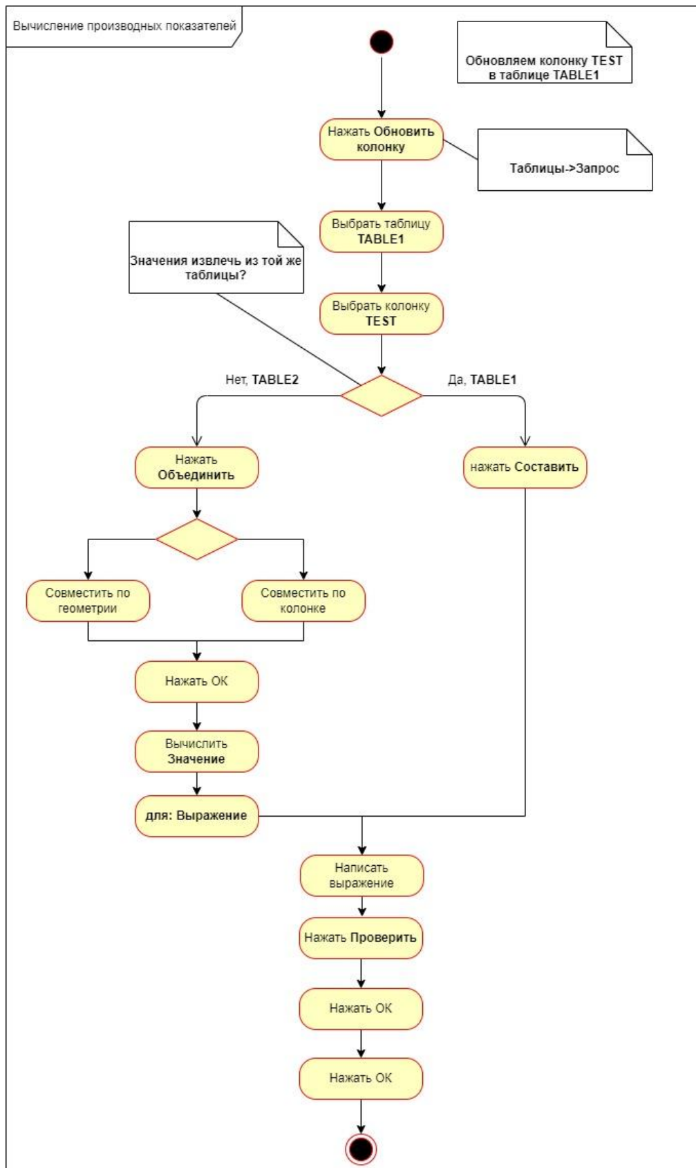
Рисунок 82 – Обновление колонки
